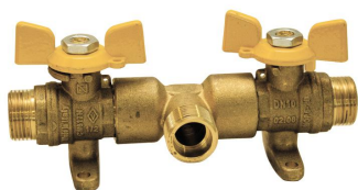
Válvulas de Esfera Gás Coletor Duplo
